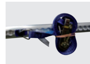
S080714343 Zurrgurt m. Fitting 800 daN Länge 3,5m
