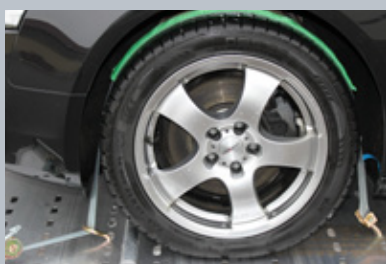
3-Punkt Verzurrung über Kässbohrer-Lochung
