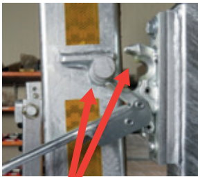
Schmierstellen
